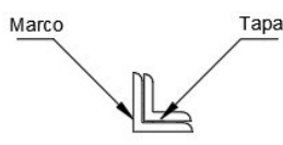
PERFIL TIPO 3 Angulo 1-1/4" con 1"
