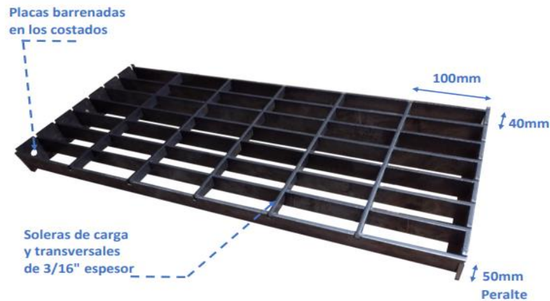
ESCALONES DE REJILLA Serie RJ-10040
